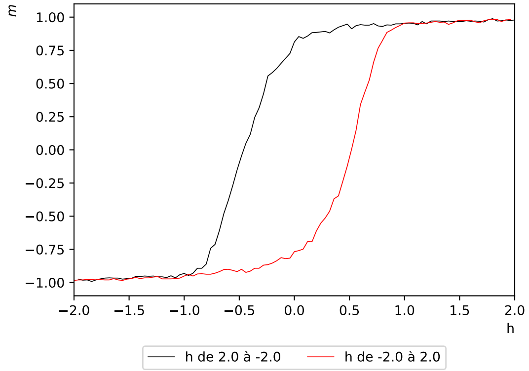
Hystérésis de l'aimantation - réseau de taille L=32 - champ magnétique d'amplitude h=2 à T=2.5
